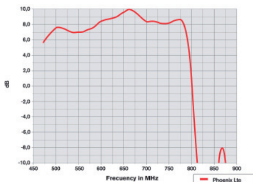
Curva de ganancia Phoenix Lte
