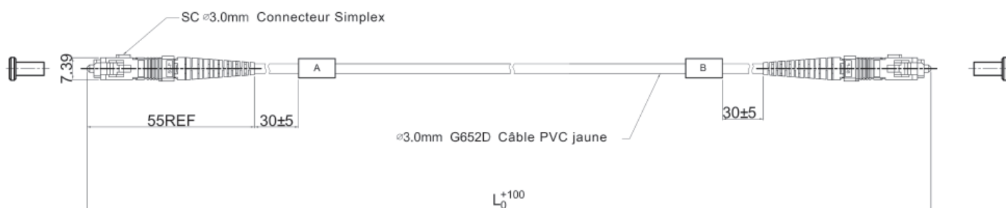
Série PCFAPC-S - dimensions en mm
