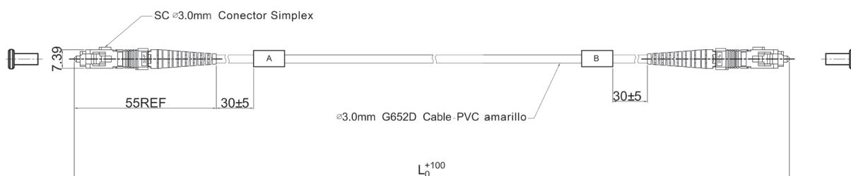
Serie PCFAPC-S - dimensiones en mm
