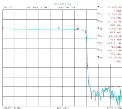
Graphiques de pertes d'insertion
