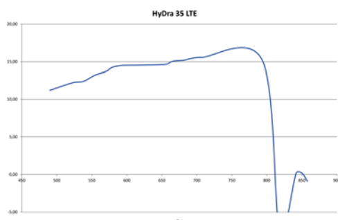
Courbe de gain HyDra 35 Lte
